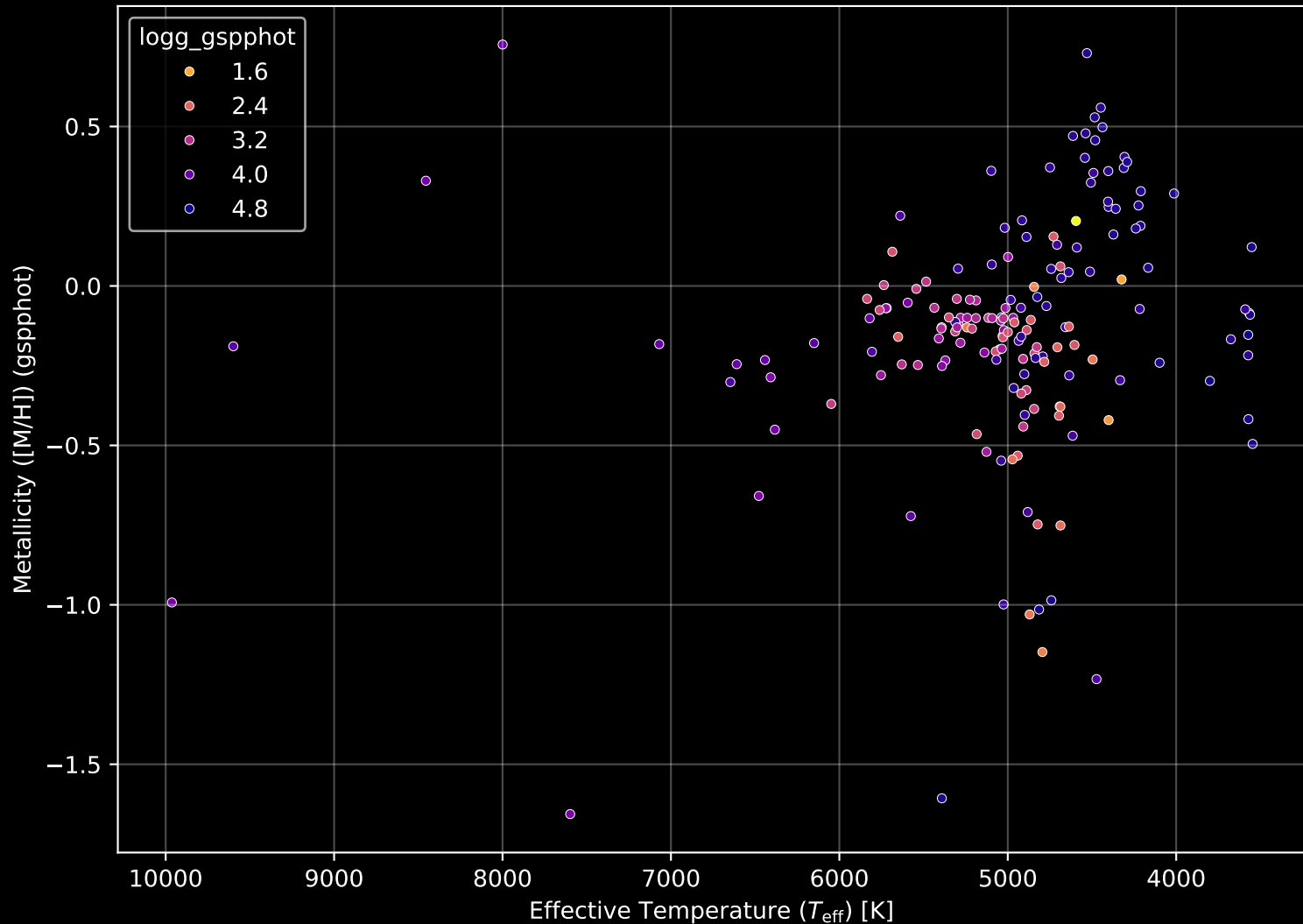
APOGEE DR17 Field: [K2_C6_331+50_btx] Stellar Population Parameters (n= 171)
